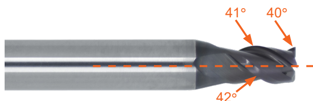
不等リード Unequal helix angle
