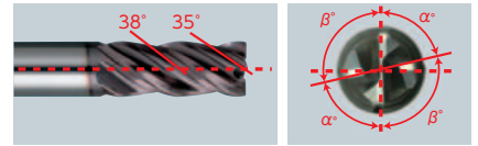
不等螺旋角 Unequal Helix Angle
